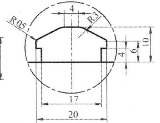
RÉSZLET C 2:1
