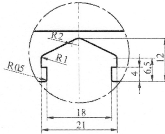
RÉSZLET B 2:1
